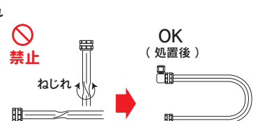
例2) 曲げたときのねじれ
