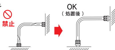
例1) 配管時のホースのねじれ
